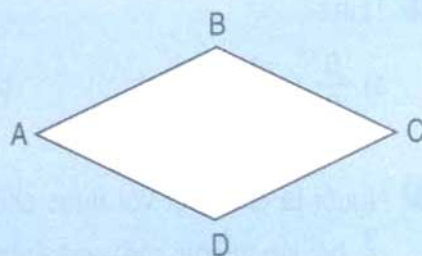
Hình thoi ABCD
