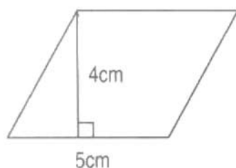
Hình bình hành
